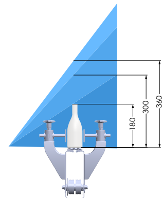
Strahlgeometrie
