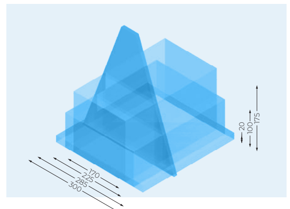
Strahlgeometrie
